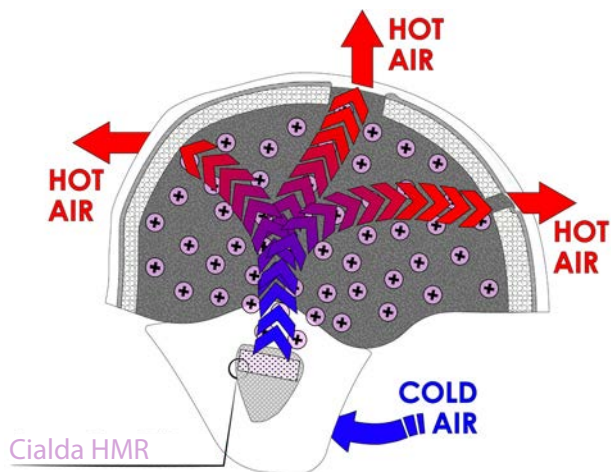
Schema di funzionamento del sistema su casco da snowboard Operating diagram of the system on the snowboard helmet
